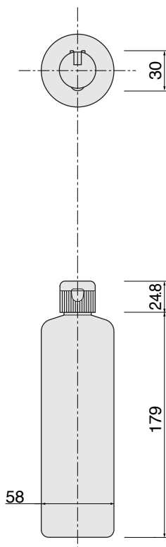
NK-400 ヒンジキャップNO.4
