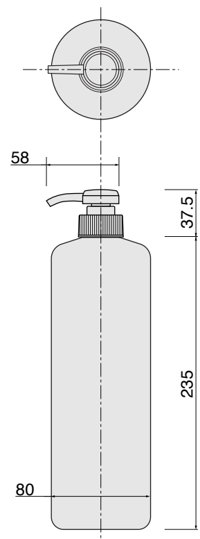
NK-1000 P-304ポンプ
