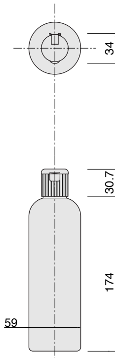
YFP-400 ヒンジキャップA
