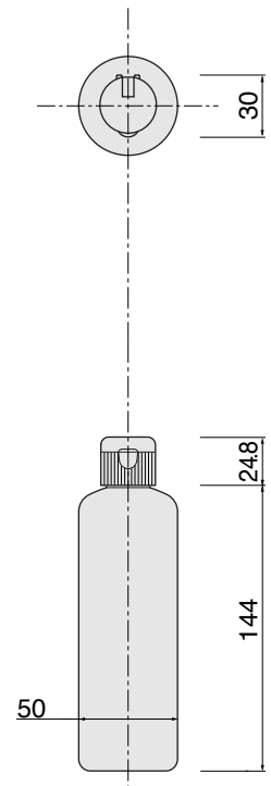
NK-240 ヒンジキャップNO.4
