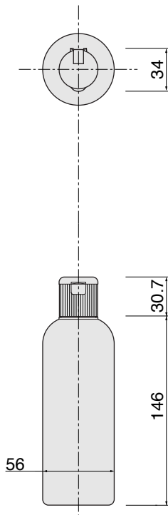
YFP-300 ヒンジキャップA
