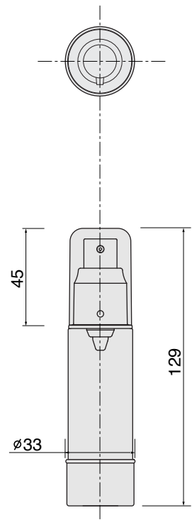
AHV24-30 銀冠 HV24ポンプ (銀冠)
