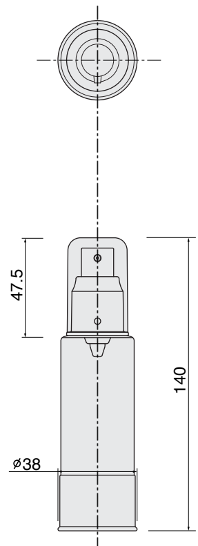
AHV24-50 銀冠 HV24ポンプ (銀冠)
