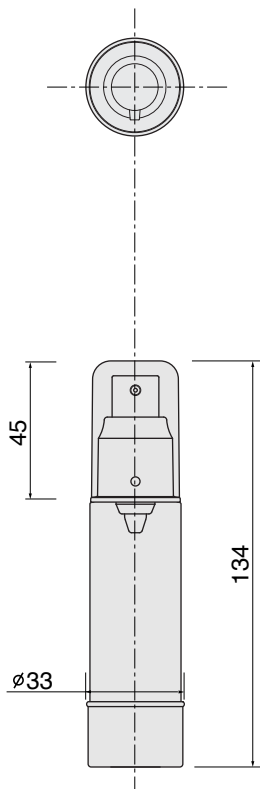
AHV24-35 銀冠 HV24ポンプ (銀冠)
