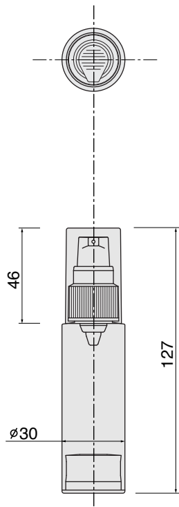
AHV24-30 樹脂 HV24ポンプ (樹脂)
