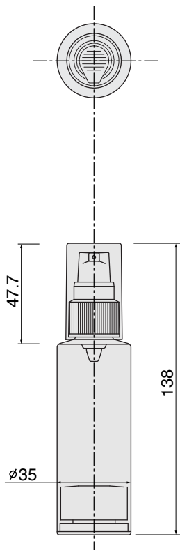
AHV24-50 樹脂 HV24ポンプ (樹脂)
